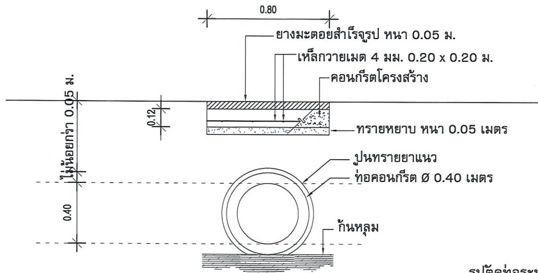
รูปตัดท่อระบายน้ำ Ø 0.40 ม. ตามขวาง
