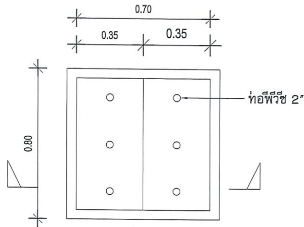
ผังพื้นบ่อพักท่อระบายน้ำ
