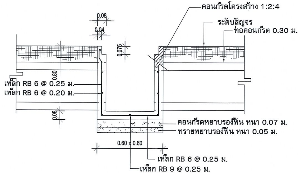
รูปตัดบ่อพักท่อระบายน้ำ
